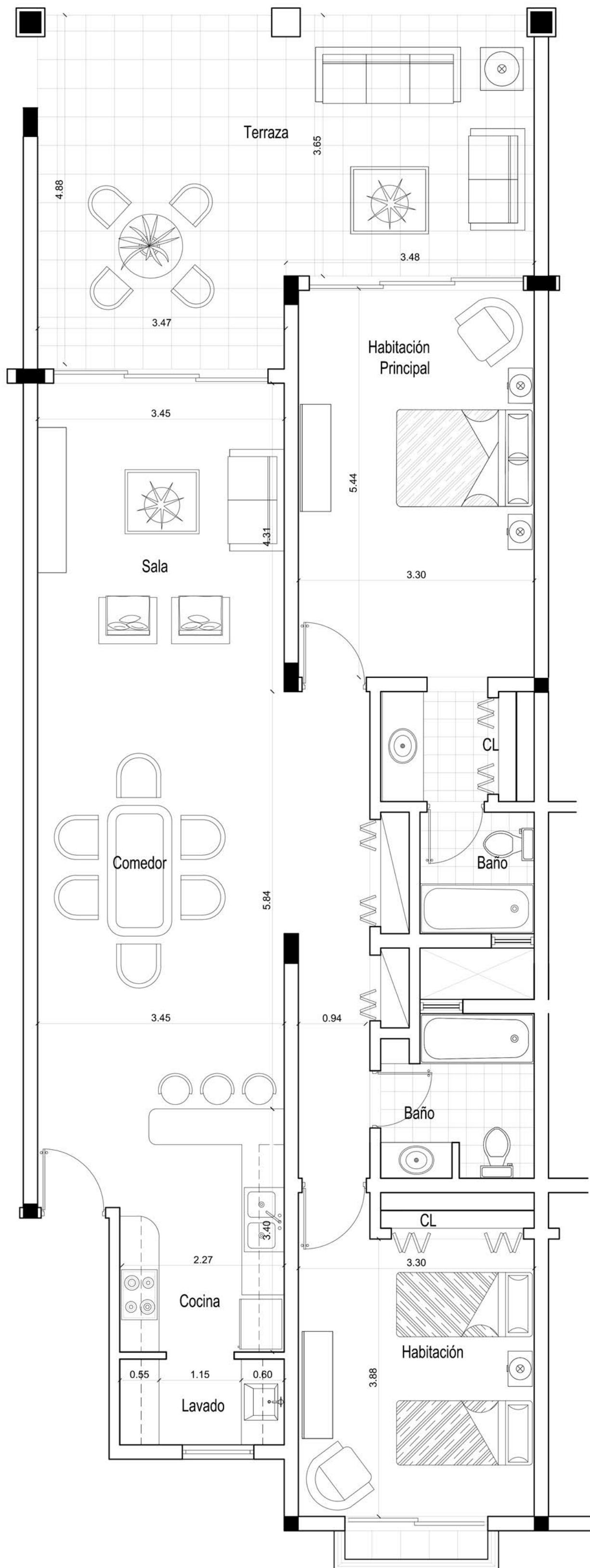
1 PLANTA AMUEBLADA ESC. 1:50
